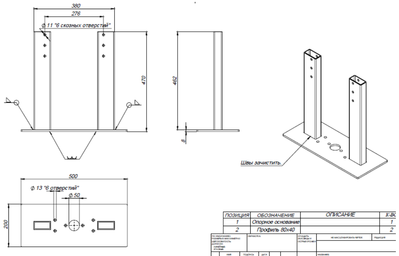
Рисунок 3 – Монтаж устройства
