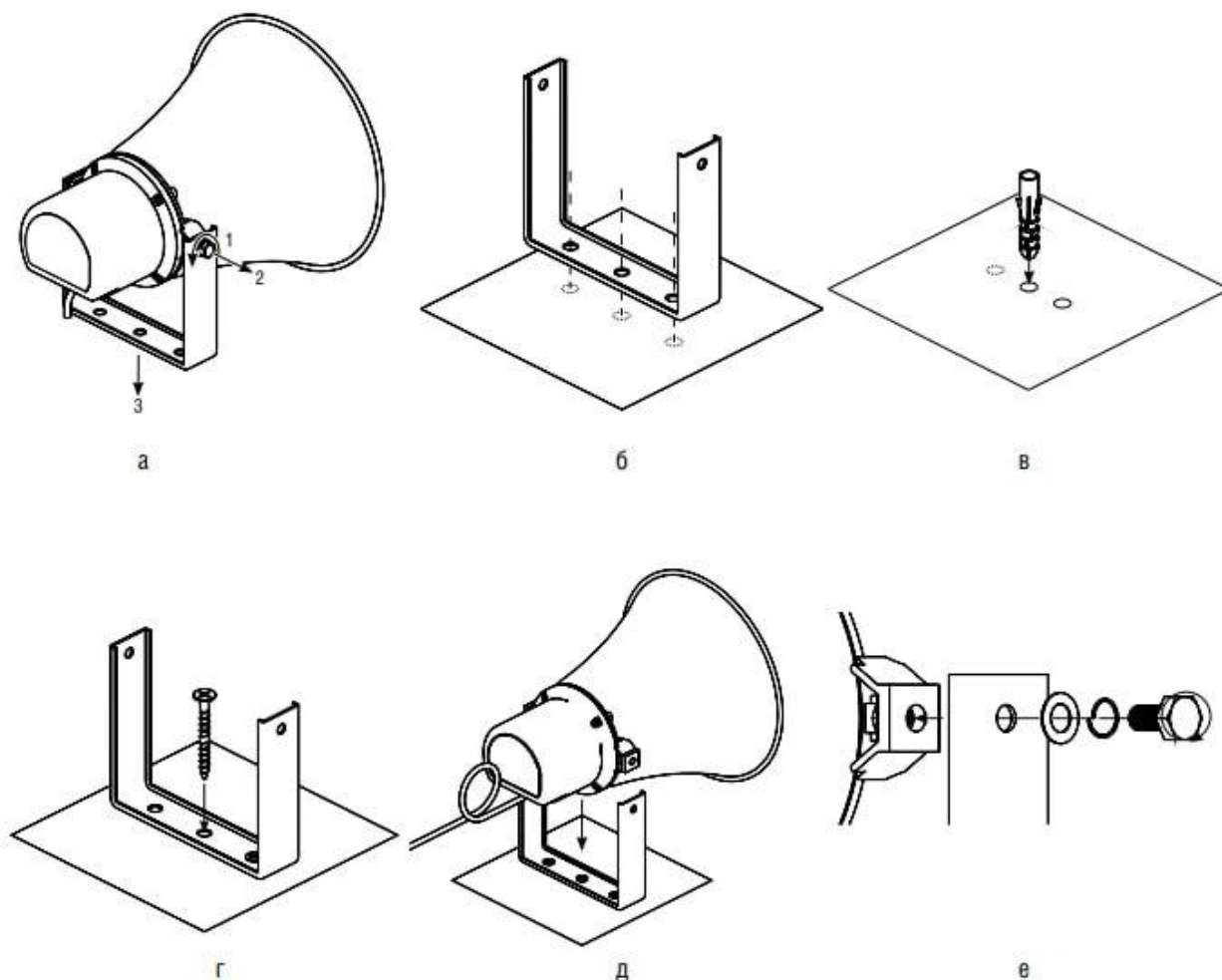
Рисунок 5 – Монтаж изделия
